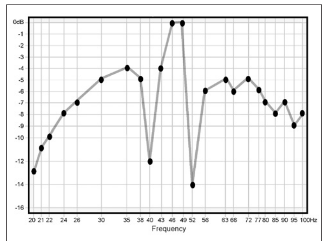
Abbildung 19. Zwei Resonanzspitzen
