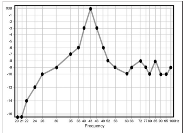
Abbildung 15. Einzelne Resonanzspitze
