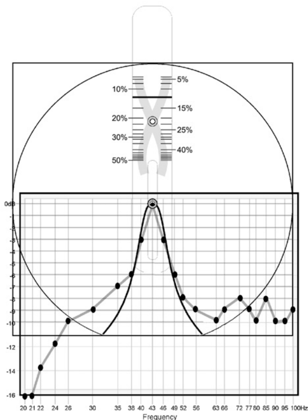
Abbildung 14. Bandbreitenschablone richtig eingestellt
