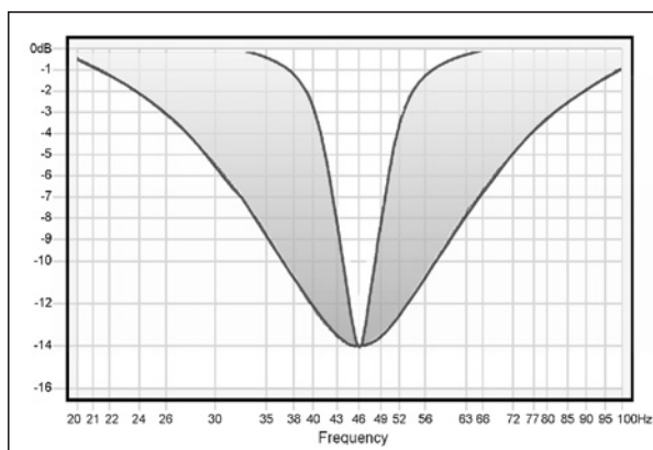
Abbildung 11. Auswirkung der einstellbaren Bandbreite
