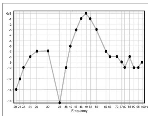
Abbildung 17. Frequenzeinbruch nach oder vor einer Resonanzspitze
